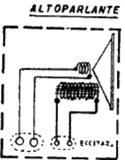
MARCONI (COMPAGNIA ITALIANA) - Mod. 1183 e mod. 1184 SERIE RICEVITORI PROFESSIONALI - Gamma onde medie intera (da 187 a 580 m) e sette gamme onde corte-cortissime (da 54,35 a 13,5 m).
