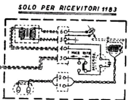
MARCONI (COMPAGNIA ITALIANA) - Mod. 1183 e mod. 1184 SERIE RICEVITORI PROFESSIONALI - Gamma onde medie intera (da 187 a 580 m) e sette gamme onde corte-cortissime (da 54,35 a 13,5 m).
